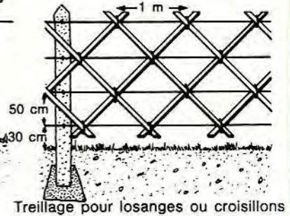
Treillage pour losanges ou croisillons
