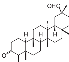
friedelan-3-on-29-al
