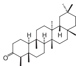
friedelin
