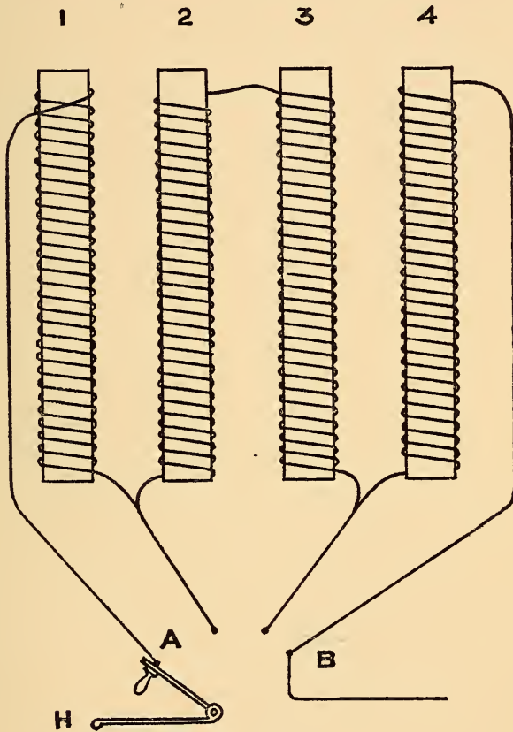
FIG. 21.—Rheostat.
