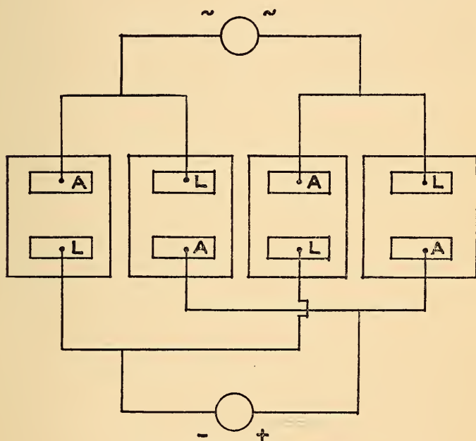
FIG. 15.—Aluminum cell rectifier.
